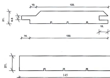
Planche bardage rabotée 4 faces
